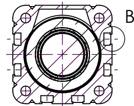
PRZEKRÓJ A-A
