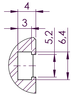
SZCZEGÓŁ B
